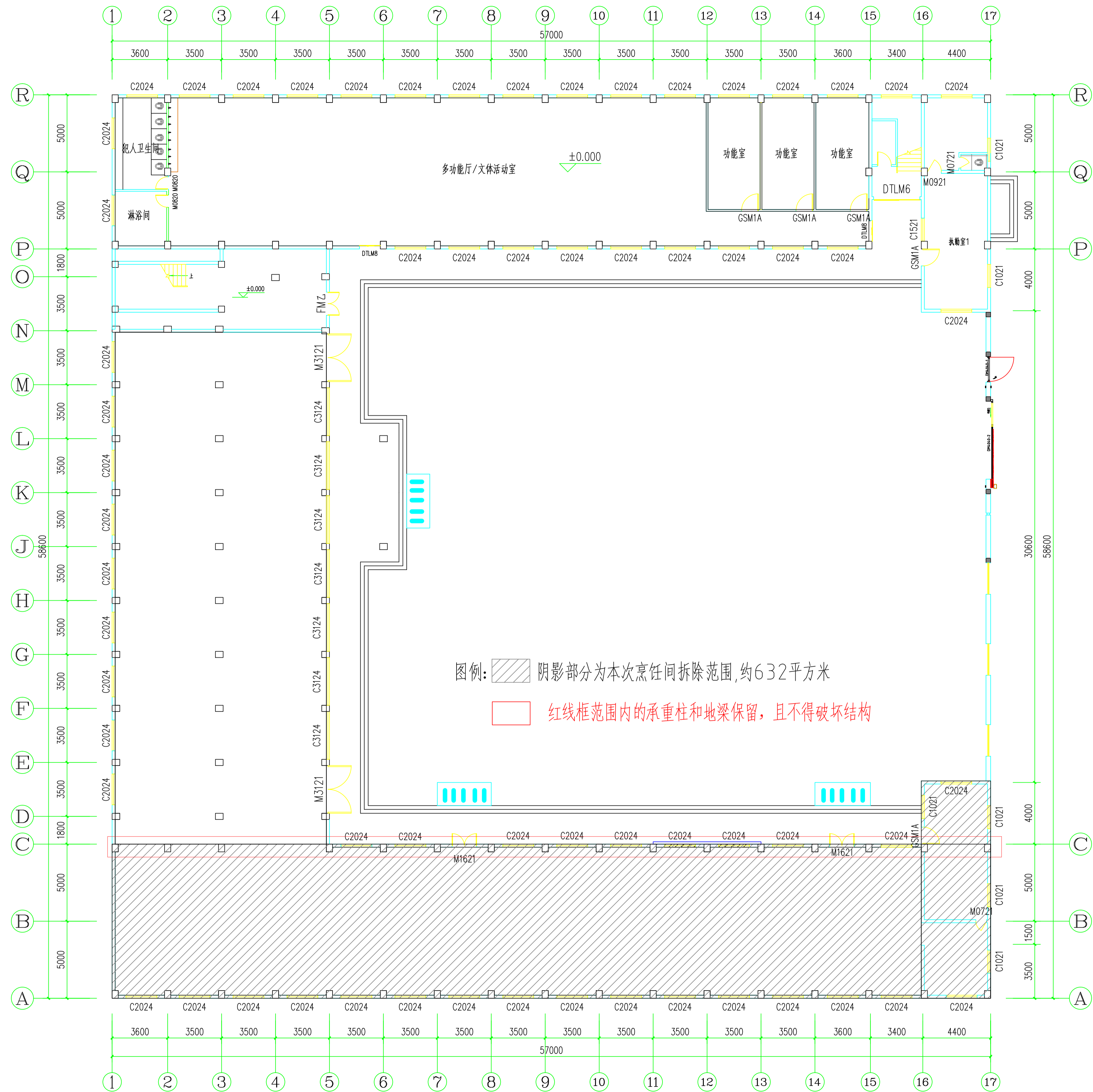
原伙房烹饪间拆除平面图 1:180
